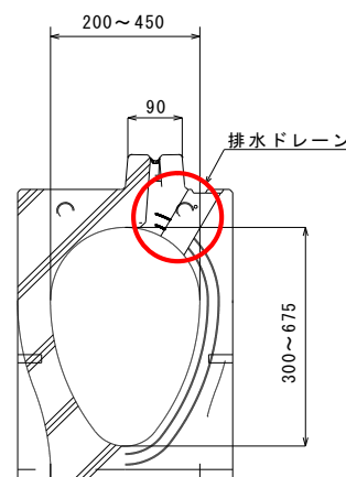
図-1 自転車に優しい側溝 径 250~500サイズ
