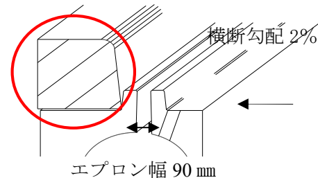
図-3 自転車に優しい側溝
