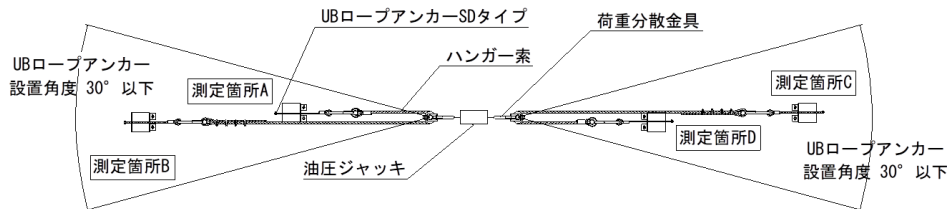
図-1 アンカー、分散金具設置図
