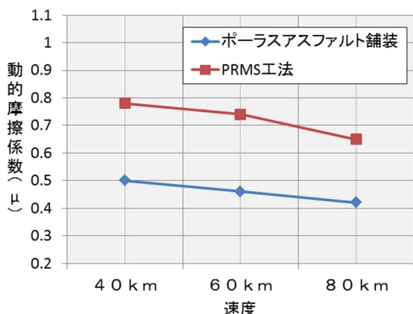
図-3 DF テスターによる測定値
