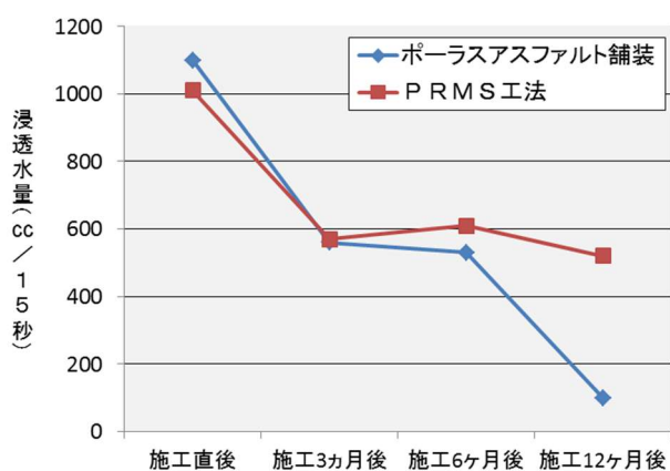
図-5 現場透水量の経時変化
