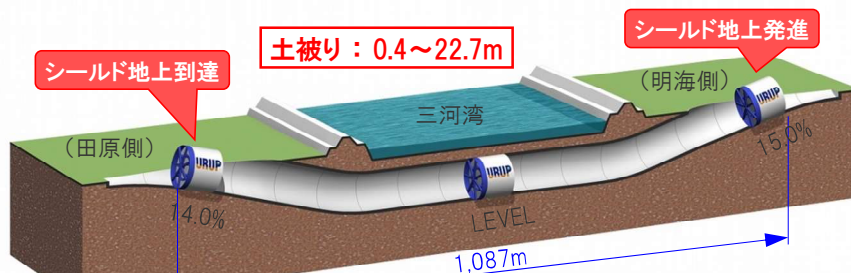
施工概要図
