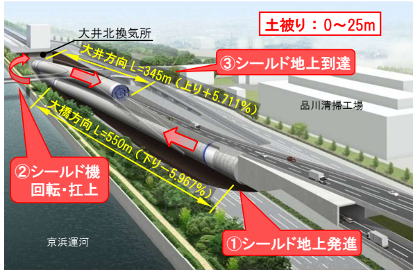
施工概要図
