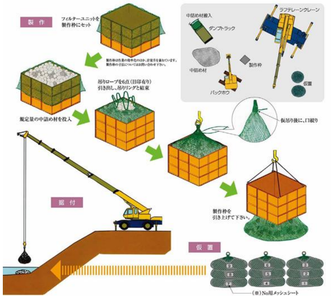
図3 エコグリーンの施工手順
